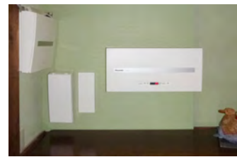
正面にあるのが、パワーコンディショナです。太陽光で発電した直流電流を家庭で使える交流に変換します。現在の発電量が表示されます。左には、電力検出ユニットが設置しており、データをエネルギーモニターに送信しています。
